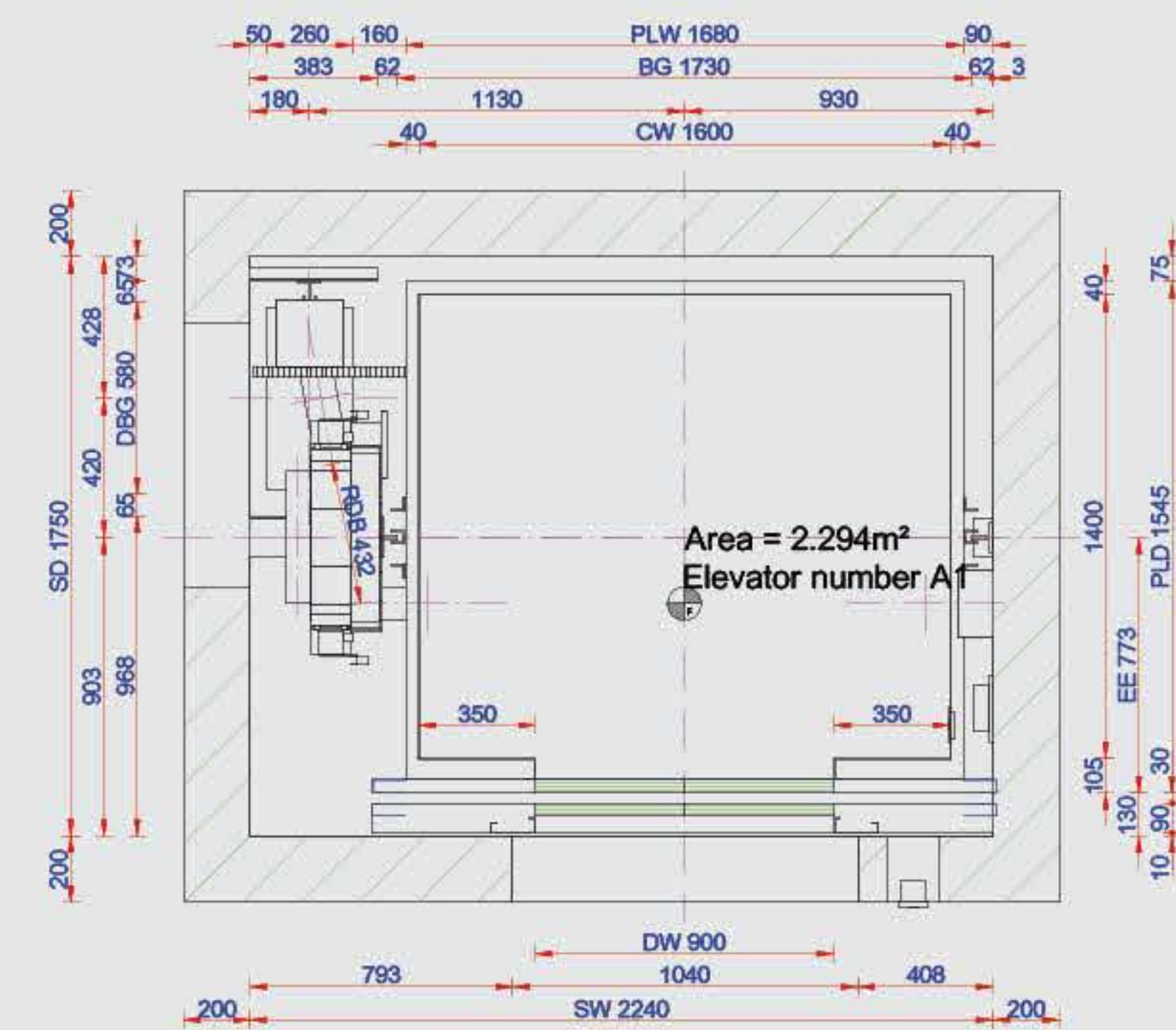
Plan Scale: 1:20
