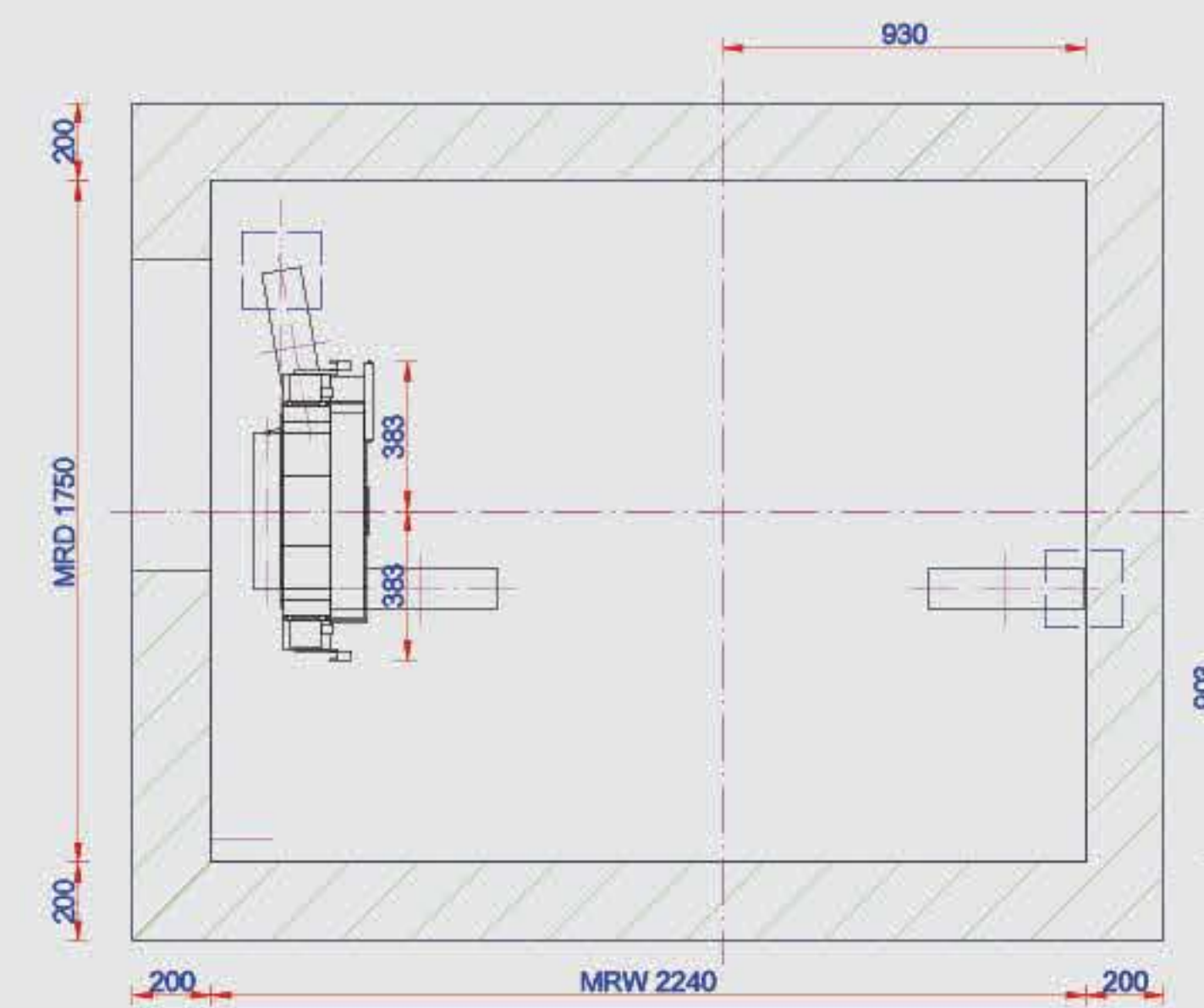
Machine room Scale: 1:20
